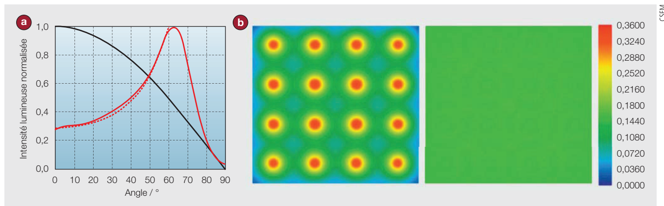
Figure 5 a) Distributions angulaires d'intensité optimale (rouge) et lambertienne (noir). La ligne pointillée rouge montre la distribution de type cosinus cube (« batwing »). b) Distribution spatiale de luminance calculée pour un groupement de 4x4 LED avec une séparation de 25 mm dans une chambre réfléchissante. La surface émettrice est de l'ordre de 10 x 10 cm 2 . Avec des LED à profil d'émission lambertien (à gauche), on obtient des valeurs d'uniformité de luminance de 30 %, tandis qu'en utilisant des sources avec une distribution lumineuse optimale (« batwing », à droite), l'uniformité peut atteindre la valeur de 89 %.
