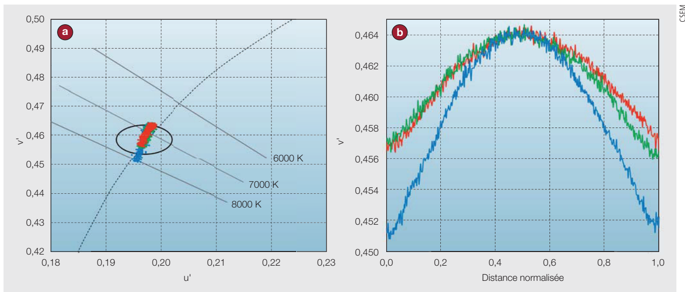
Figure 4 a) Coordonnées de couleur CIE u' v' de la lumière émise par différents points à travers la surface émettrice d'un module commercial à éclairage périphérique. Le cercle correspond au « 5-step McAdam circle ». b) Coordonnées de couleur CIE v' le long des lignes bissectrices verticale (rouge), horizontale (vert) et diagonale (bleu) de la surface du module en fonction de la distance du bord.
