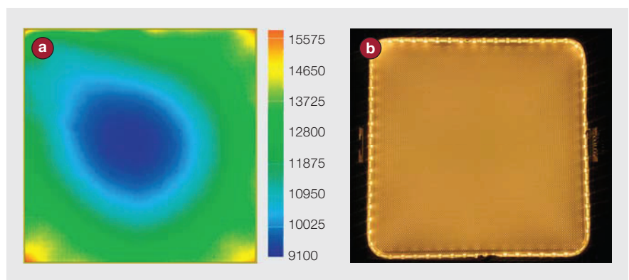
Figure 3 Module LED à éclairage périphérique (« edge-lit ») : a) Distribution spatiale de la luminance mesurée sur la surface émettrice d'un panneau LED commercial. L'uniformité est de l'ordre de 55% pour une variation de la température de couleur corrélée \Delta\text{CCT} = 2186 \text{ K} . b) Image de l'intérieur du panneau LED à éclairage périphérique testé.
